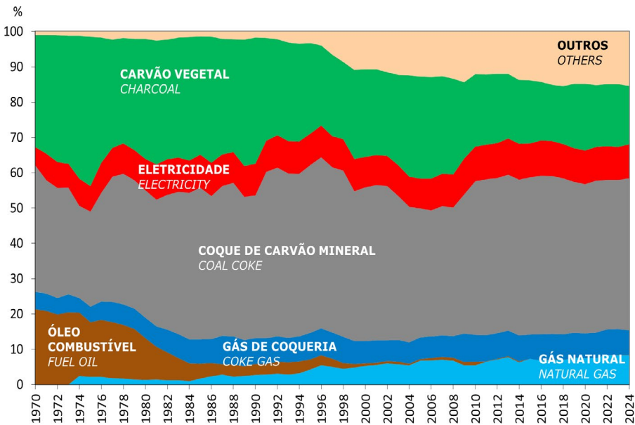
Gráfico 3.7 – Estrutura do Consumo no Setor Ferro-gusa e Aço Chart 3.7 – Pig-Iron and Steel Sector Energy Consumption
