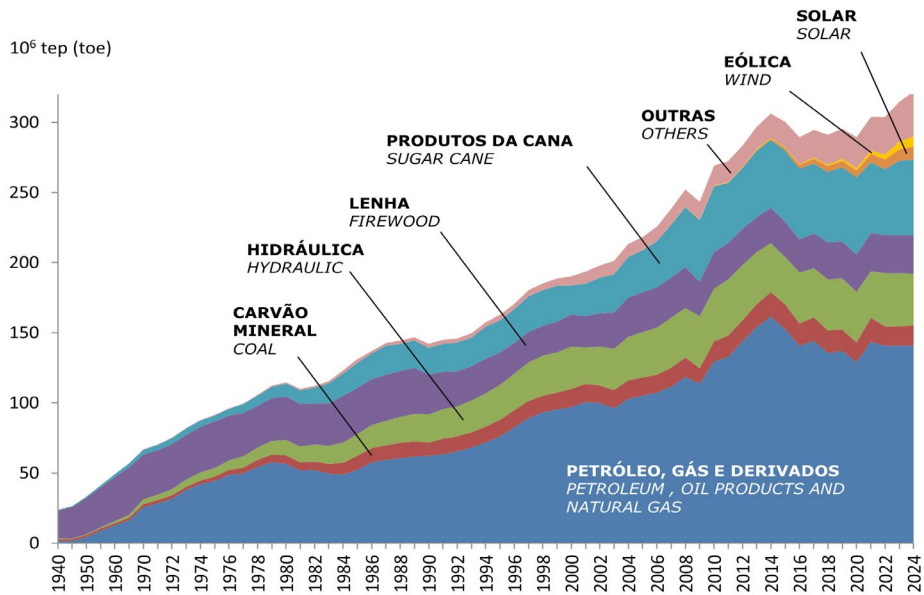
Gráfico 1.13.a – Oferta Interna de Energia
