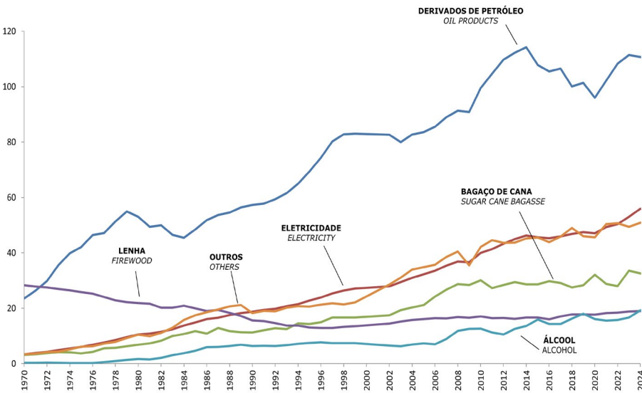
Gráfico 1.4.a – Consumo Final por Fonte Chart 1.4.a – Final Energy Consumption
