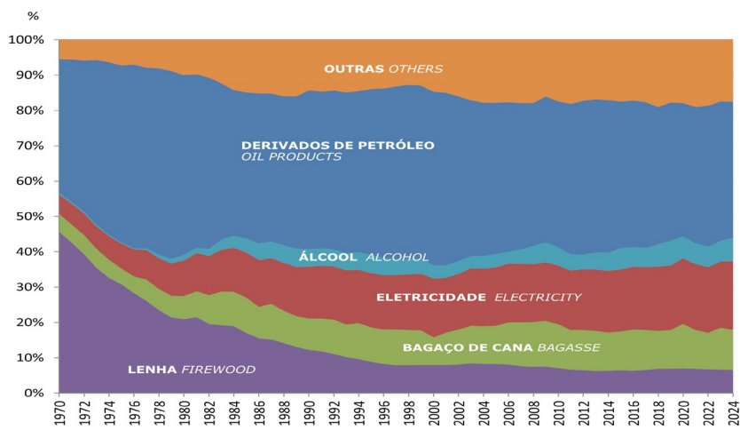
Gráfico 1.4.b – Consumo Final por Fonte Chart 1.4.b – Final Energy Consumption
